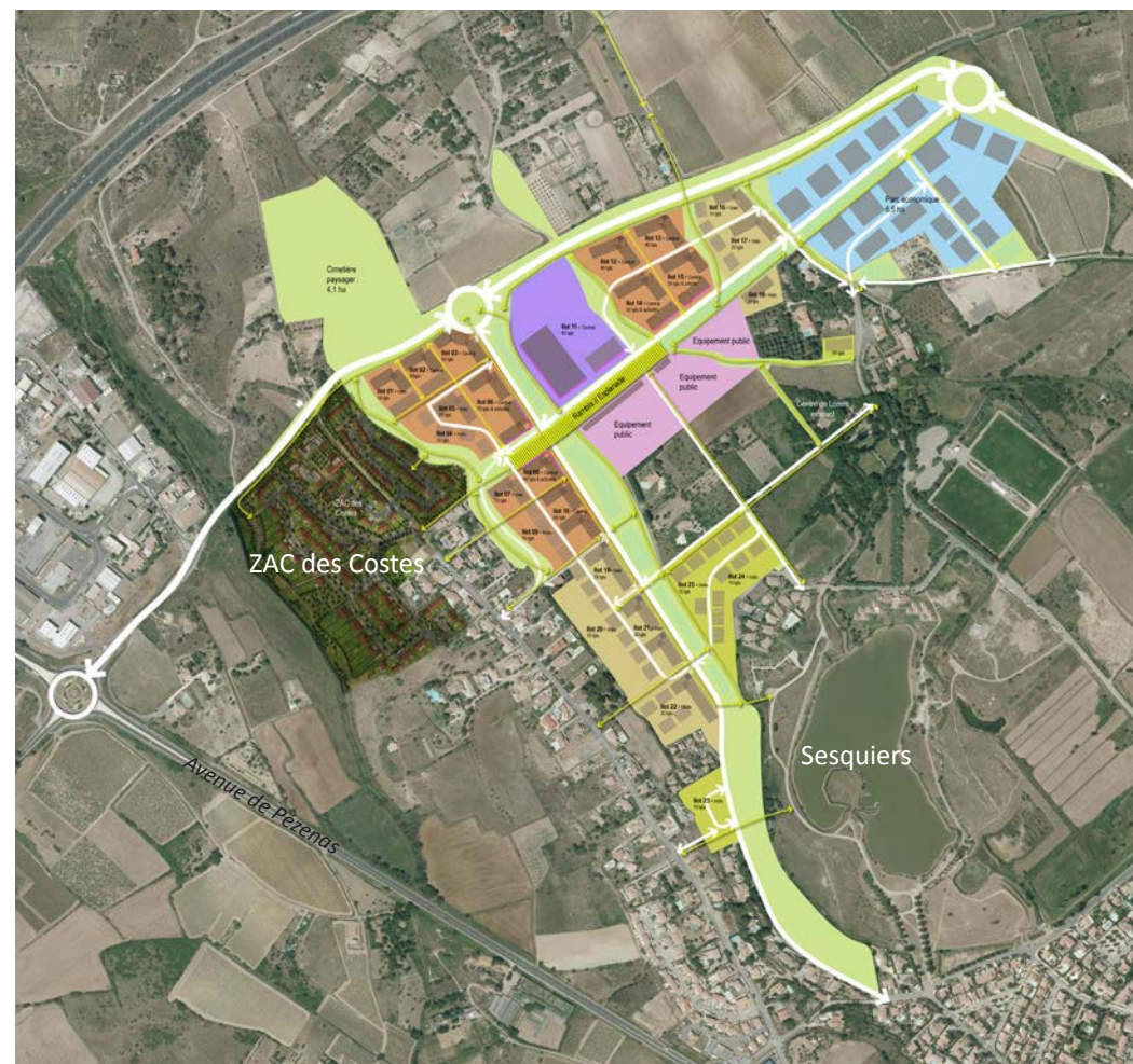
OAP Nord Sesquiers : Plan schématique des prescriptions et intentions d'aménagement.
